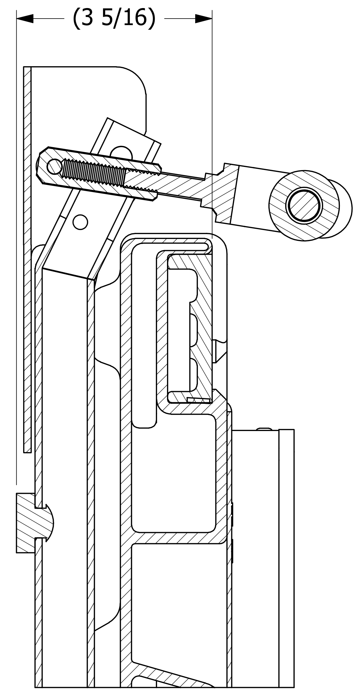
SECTION A-A SCALE 1:1
