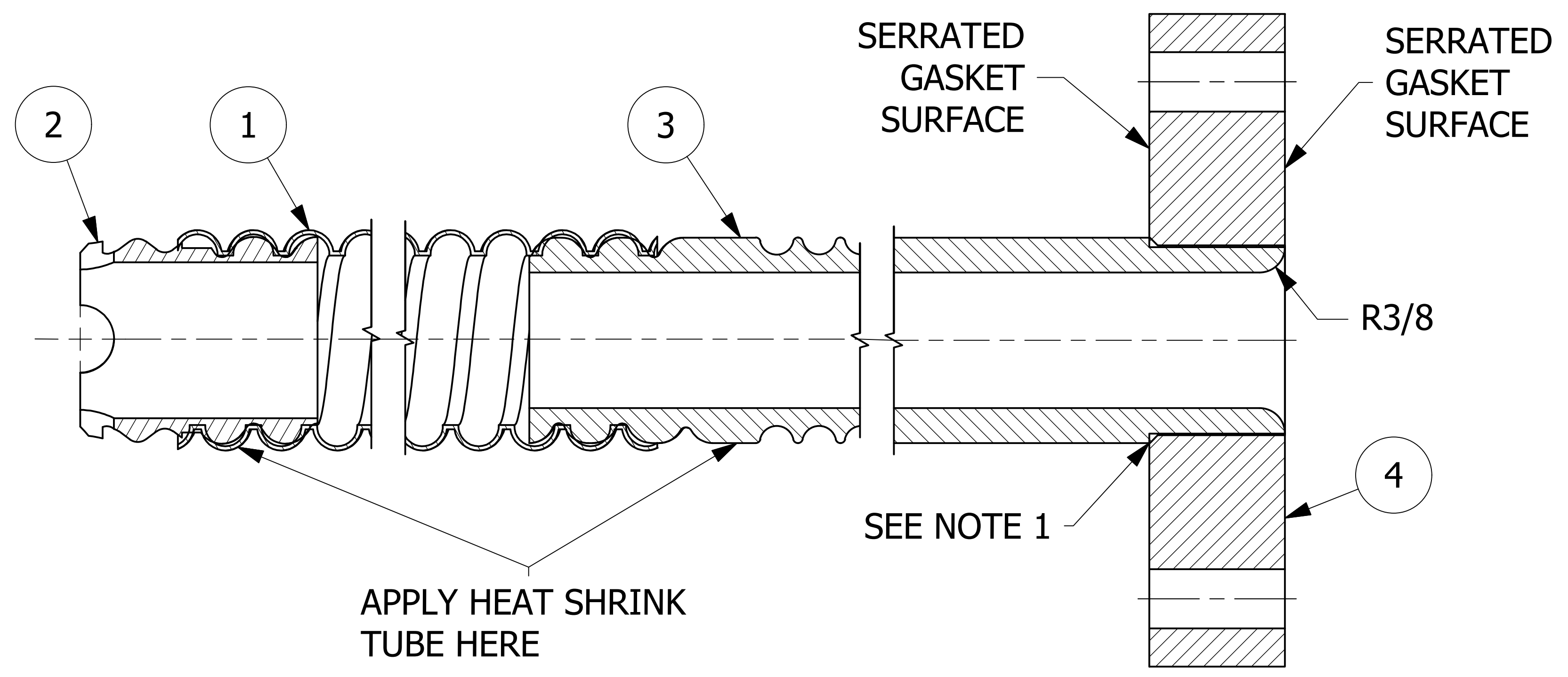
SECTION A-A
